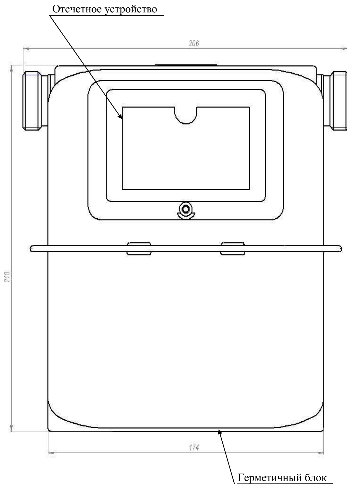
Рисунок 2 - Счетчик газа бытовой СГБ G4-1 СИГНАЛ или СГБ G2,5-1 СИГНАЛ
