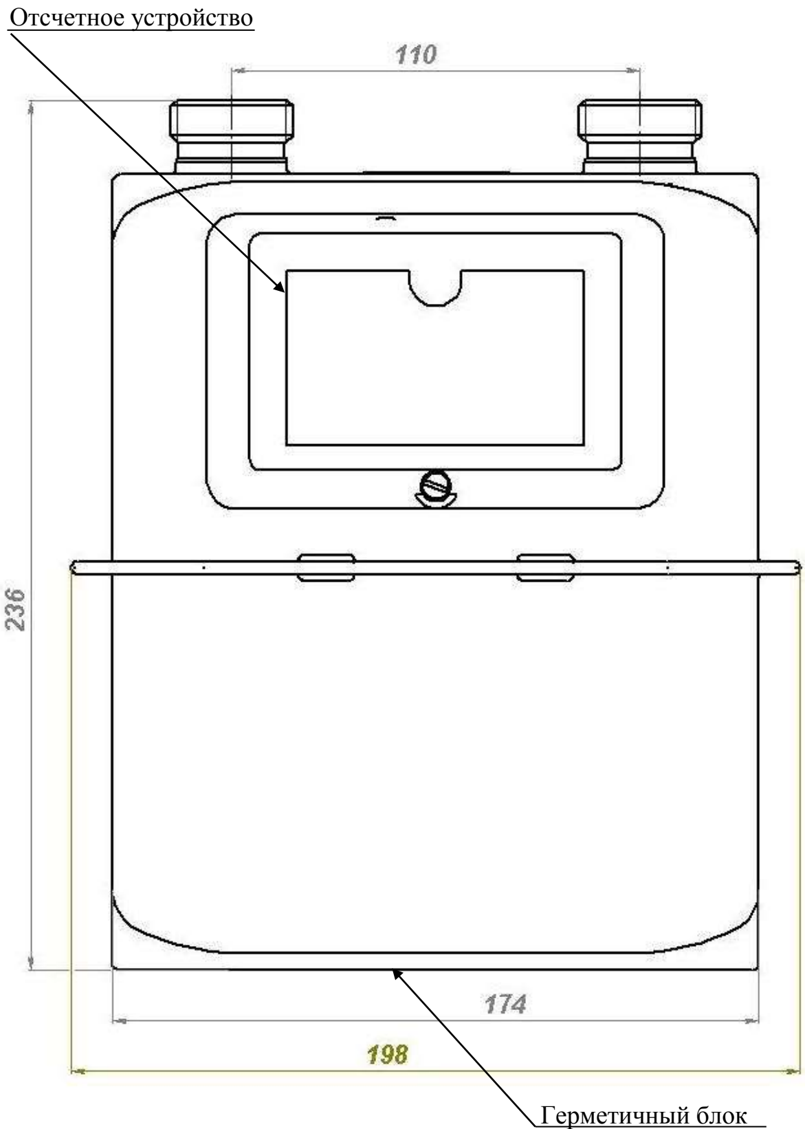
Рисунок 1 – Счетчик газа бытовой СГБ G4 СИГНАЛ или СГБ G2,5 СИГНАЛ
